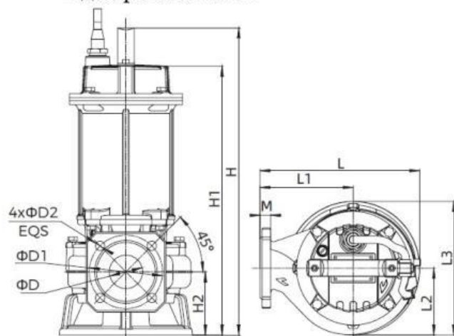
Однофазный насос
