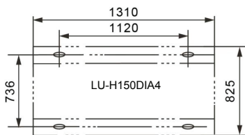
Отверстия для крепежа, 15*20мм
