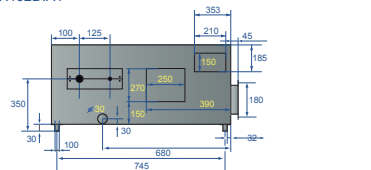
Сторона труб
