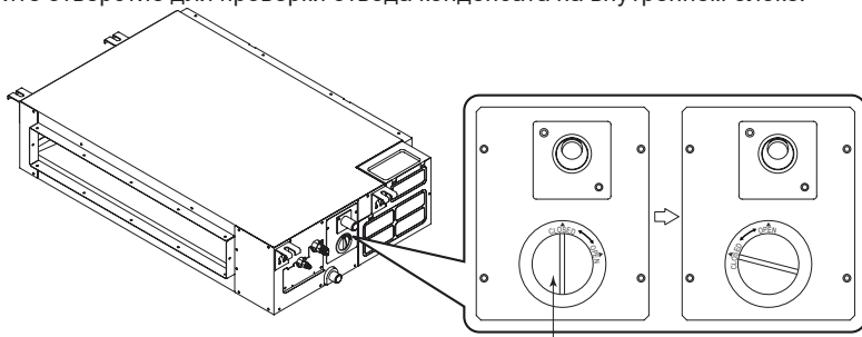
Отверстие для проверки отвода конденсата
