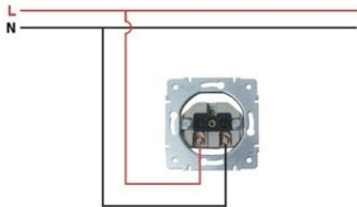
Схема подсоединения / Connection Diagram
