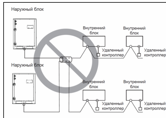
Многожильный кабель
