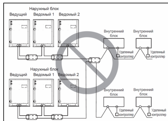
Многожильный кабель
