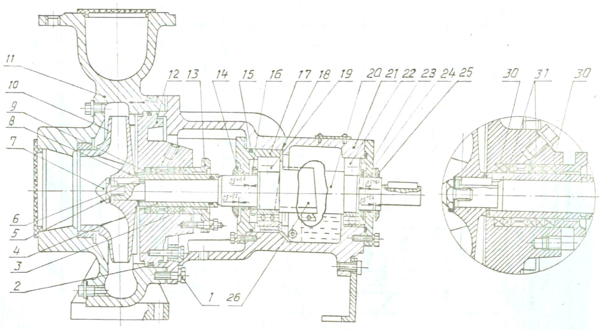
Рисунок 2 – Разрез насоса
