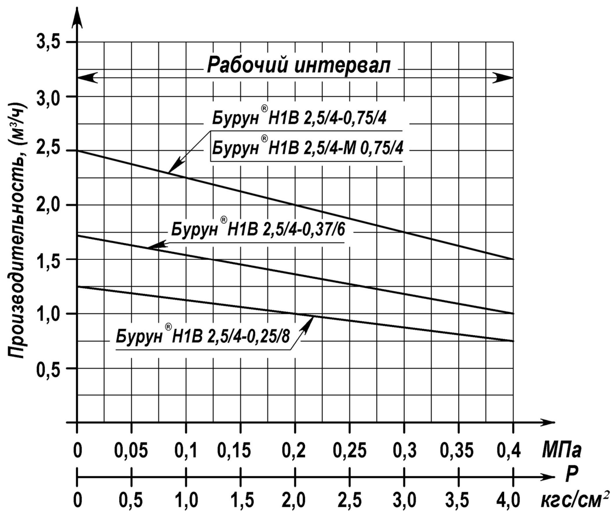
Рисунок 2 – Характеристики электронасосов
