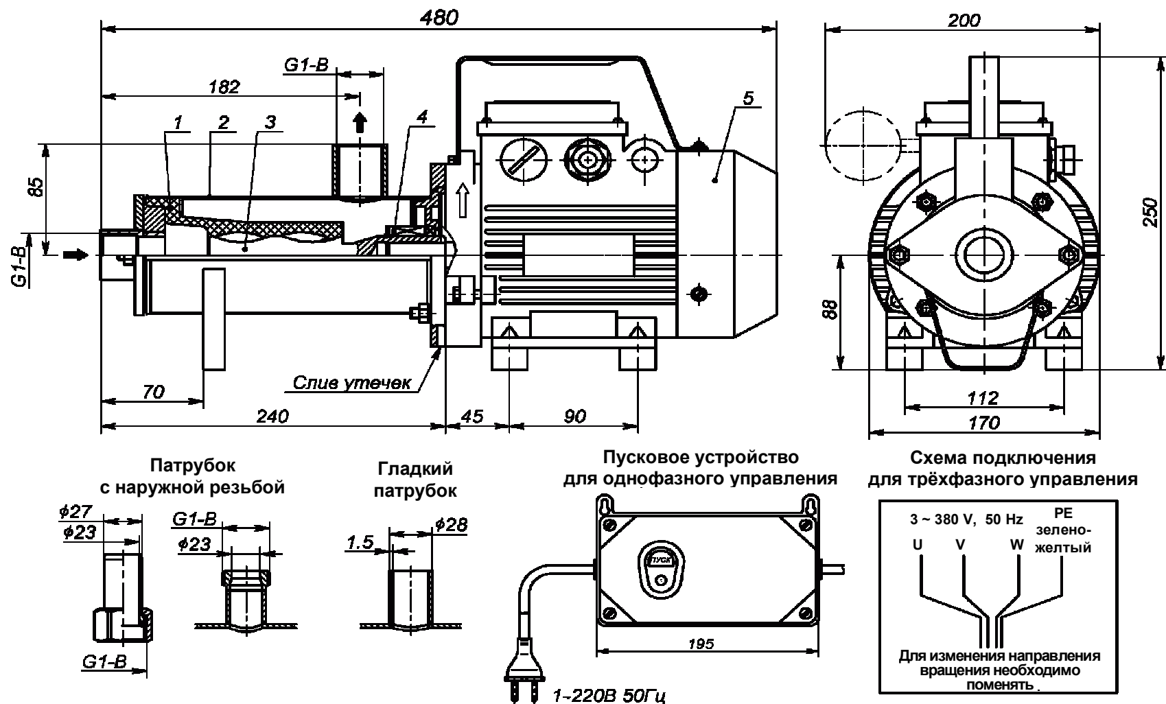
Рисунок 3 – Устройство электронасосов Бурун® CX: 0,9/4-0,25/8, 1,2/4-0,37/6, 1,8/4-0,55/4, 3,6/4-0,75/2.
