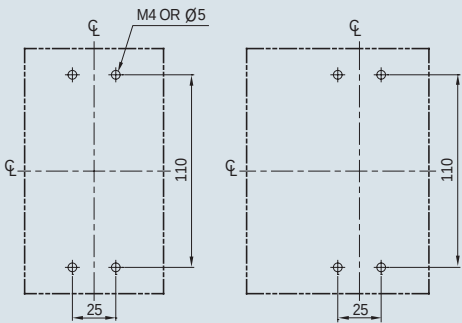
Разметка отверстий
