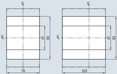
Размер выреза в передней панели
