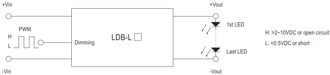
Fig-1 LDB-300L
