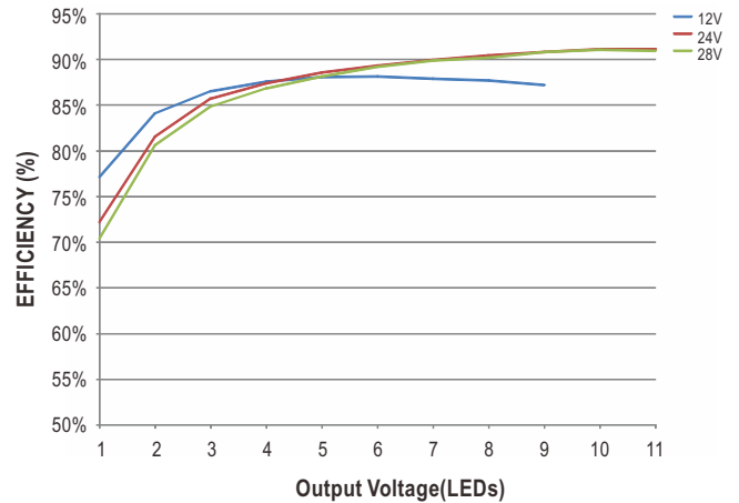
Fig-4 LDB-600L
