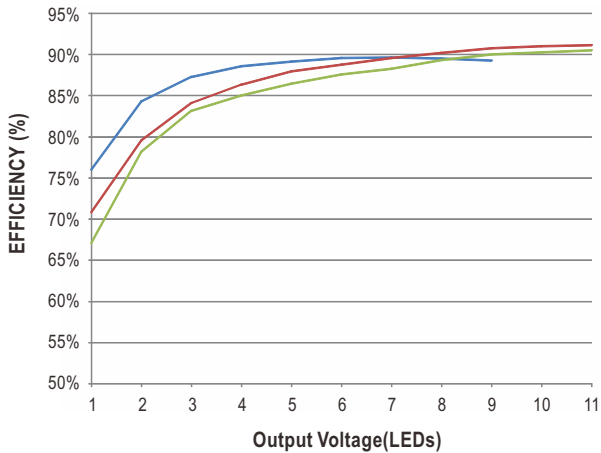
Fig-3 LDB-500L
