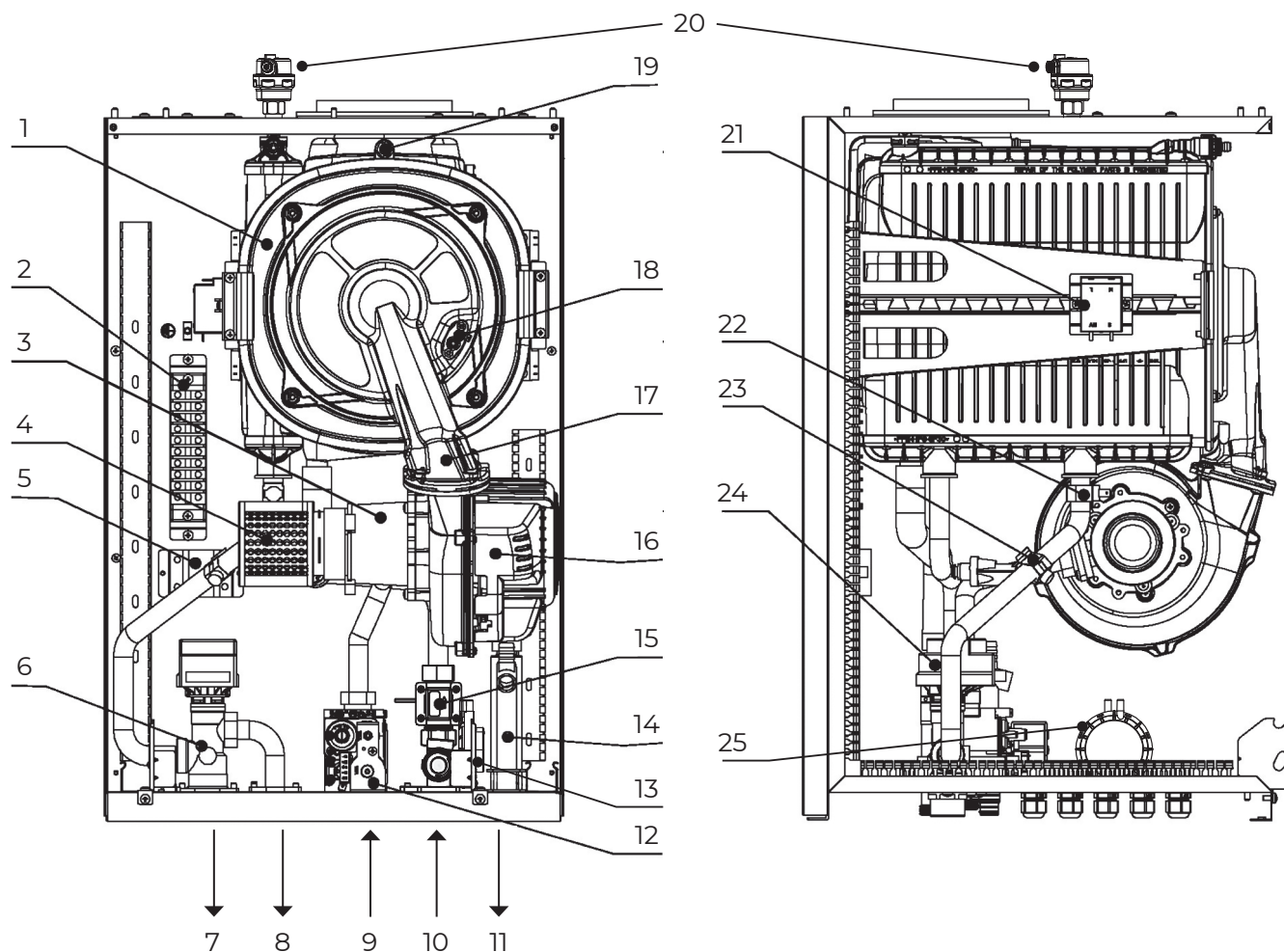
Рис. 2. Общая схема.
