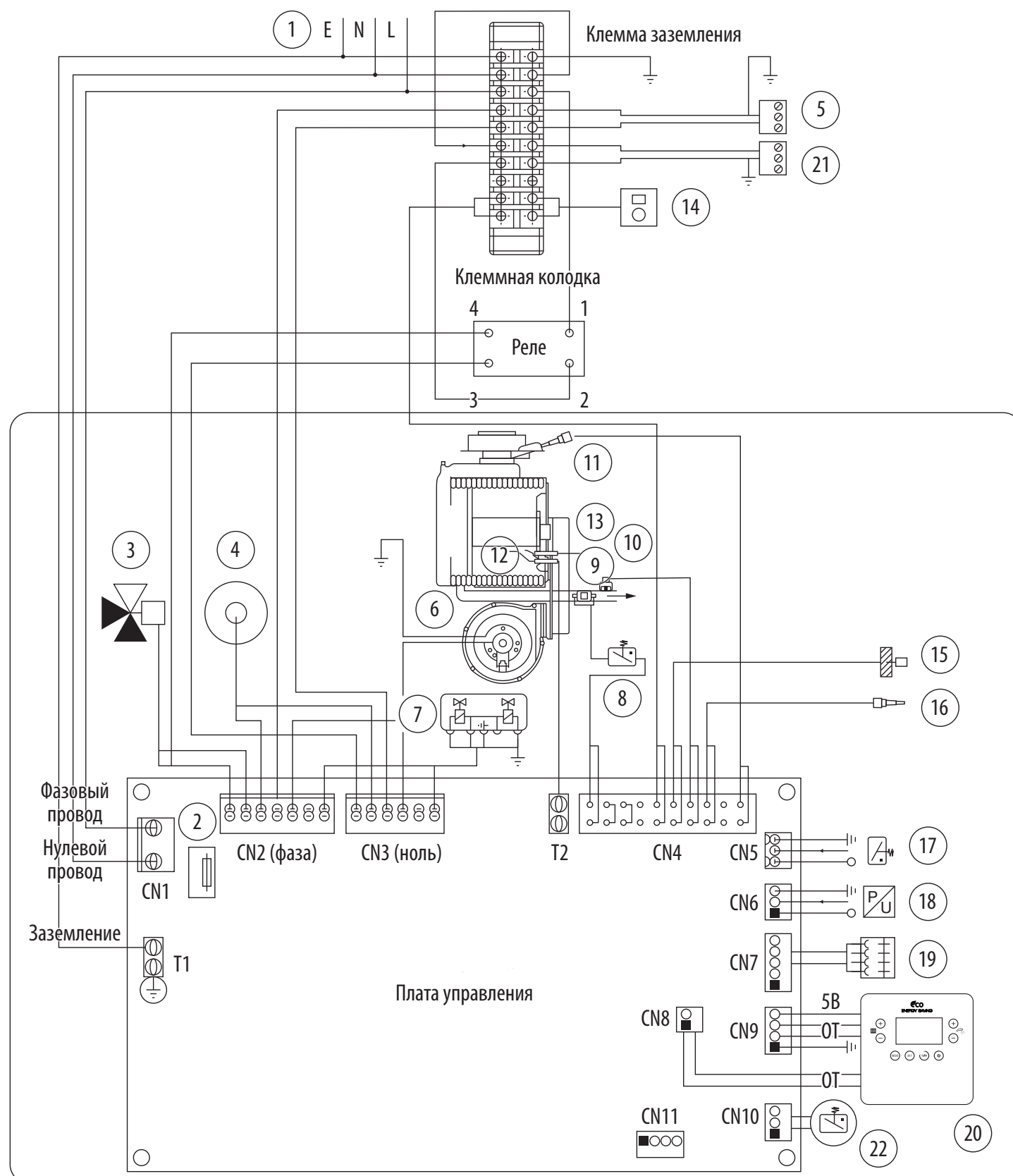
Рис. 41. Электрическая схема платы (описание на следующей странице).
