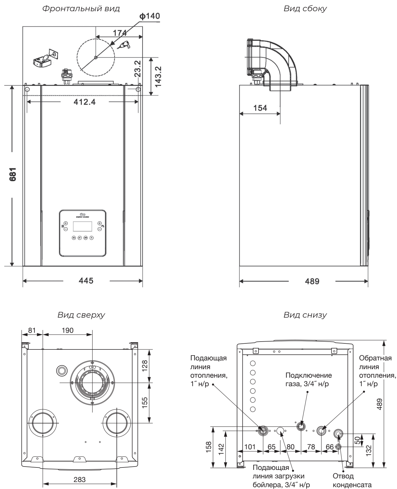
Рис. 37. Монтажные размеры.
