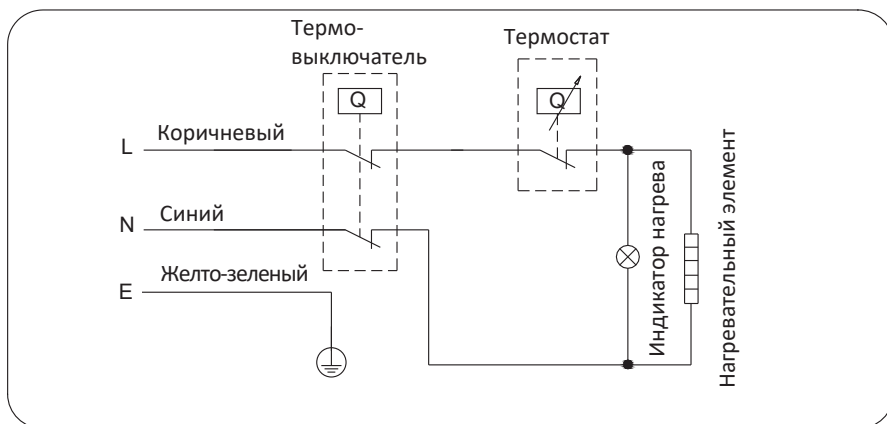
Электросхема
