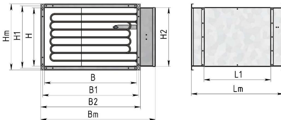
Тип 1. Клеммная коробка выступает за габариты корпуса
