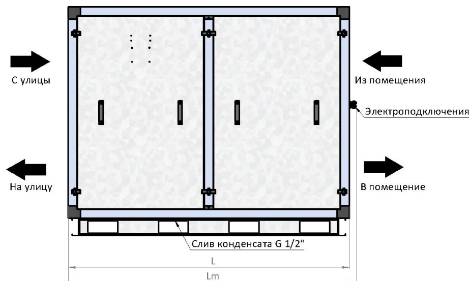
Вид спереди
