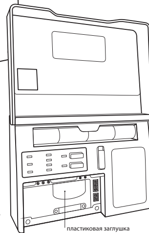
Рис.13. Вид модуля управления Neptun ProW с открытой крышкой коммутационного отсека
