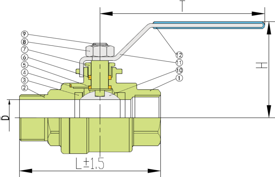
Табл.1 Размеры
