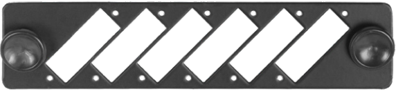
NMF-AP06DSC-P-BK до 6 двойных адаптеров SC
