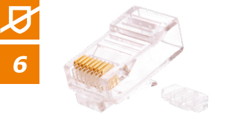
NMC-RJ88RZ50UE3-100 RJ45/8P8C, Кат,6, UTP, 50 мкд, со вставкой, универсальные ножи, круглый ввод
