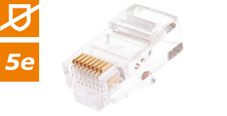
NMC-RJ88RE06UD1-100 RJ45/8P8C, Кат,5е, UTP, 6 мкд, под многожильные кабели, круглый ввод
