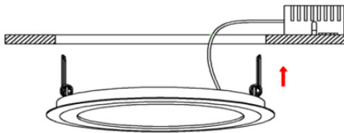
3) установка светильника
