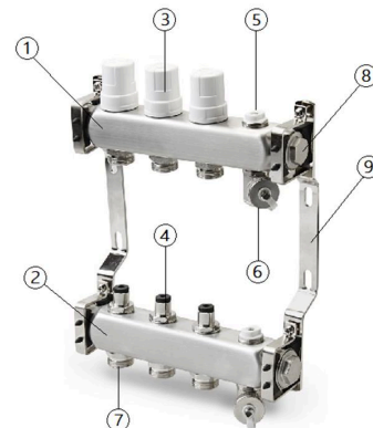
Рис. 1 Коллекторный блок с регулировочными клапанами, дренажным краном и краном Маевского, 3 вых., 1 x 3/4ЕК
