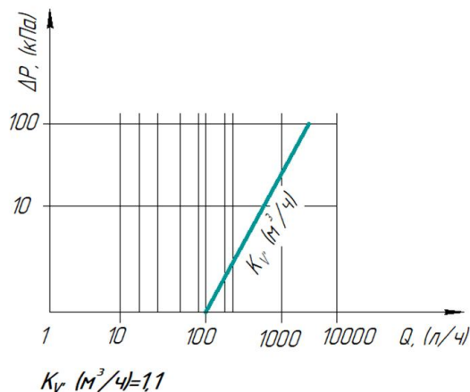
Рис. 2 Диаграмма гидравлического сопротивления балансирующего расходомера
