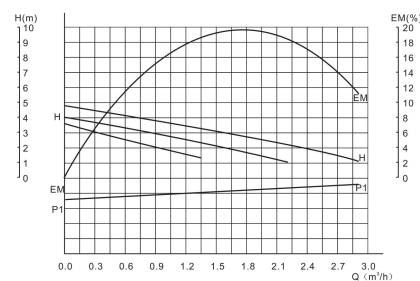
Рисунок 5 – График рабочих характеристик для серии 32/4G-180
