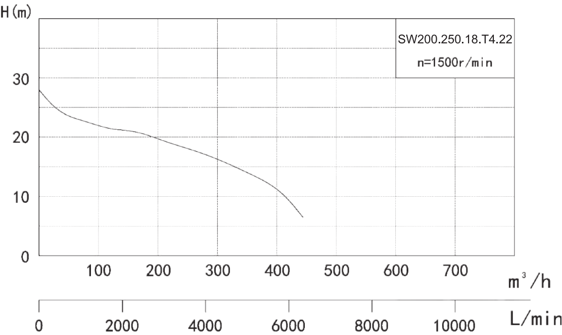
Гидравлическая кривая
