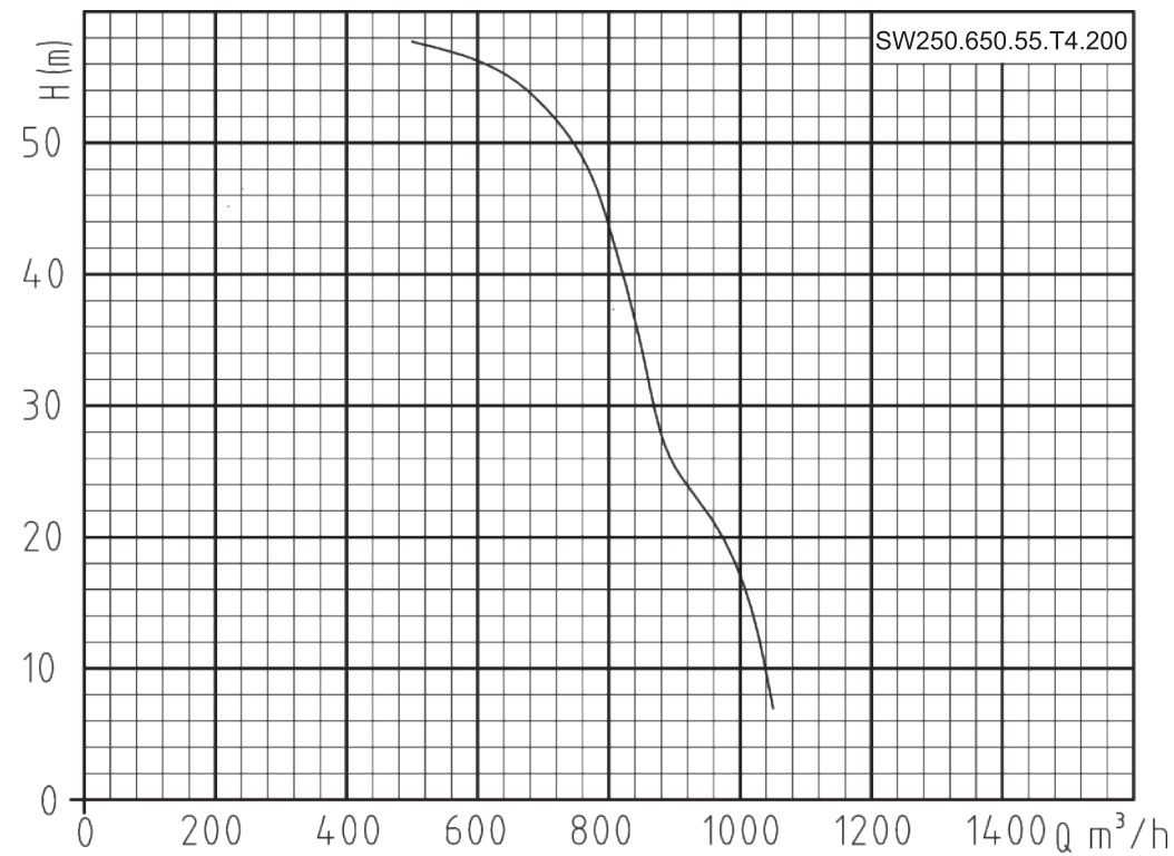
Гидравлическая кривая
