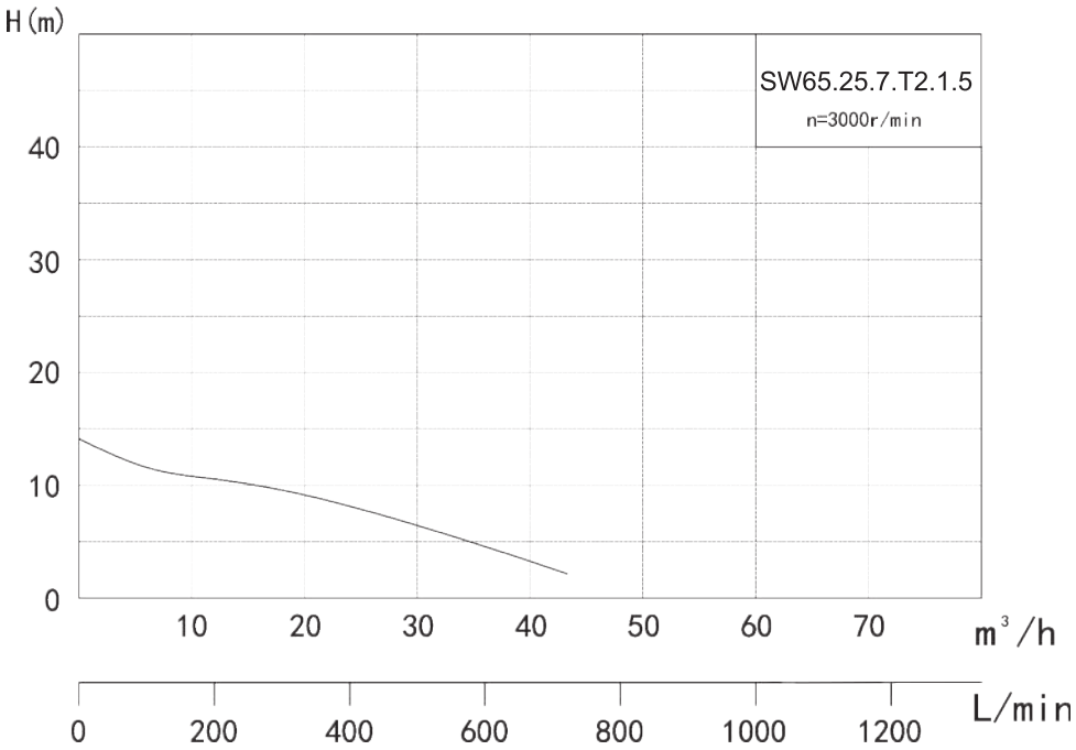
Гидравлическая кривая
