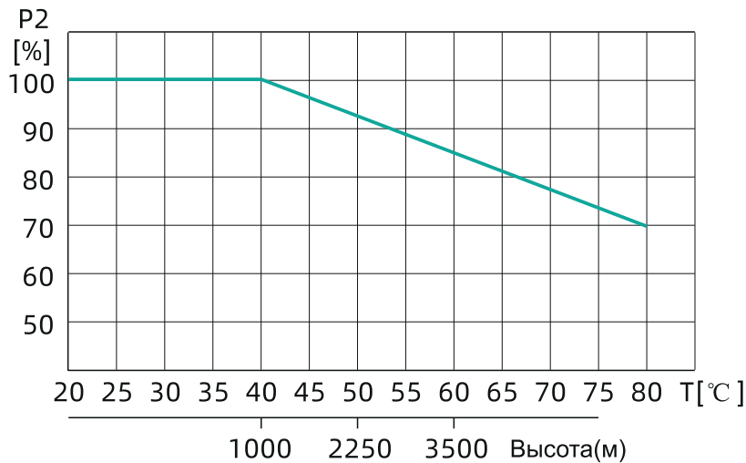
Зависимость между выходной мощностью двигателя (P2) и температурой окружающей среды
