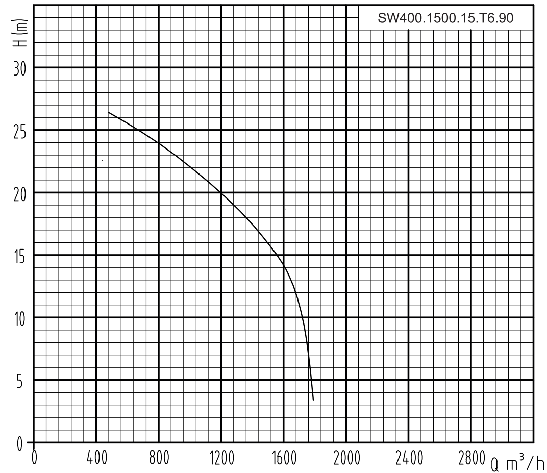
Гидравлическая кривая
