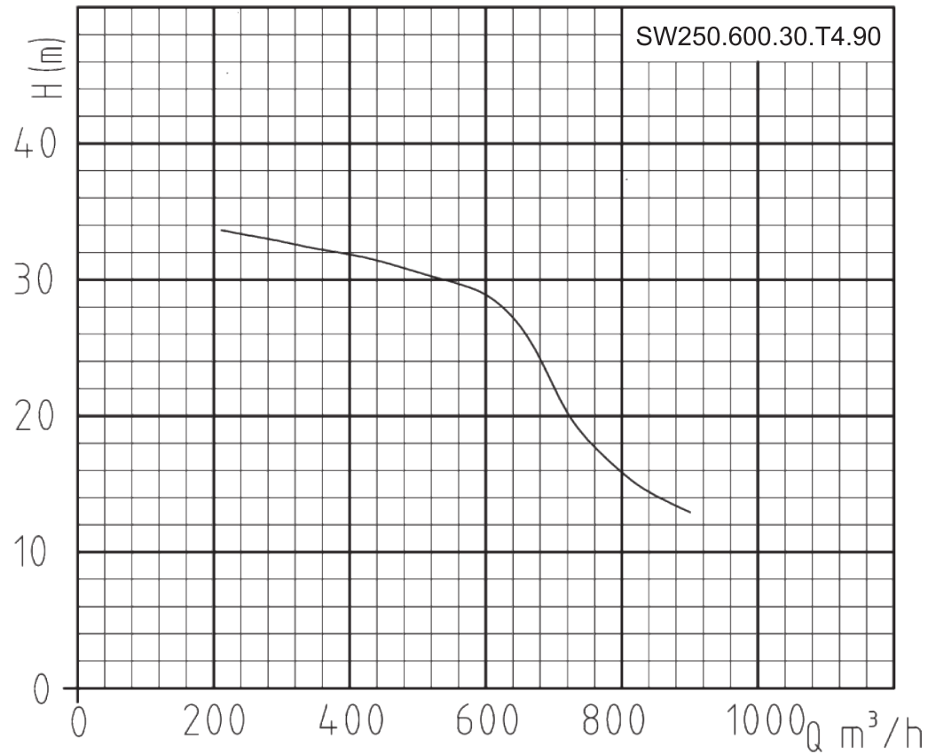
Гидравлическая кривая
