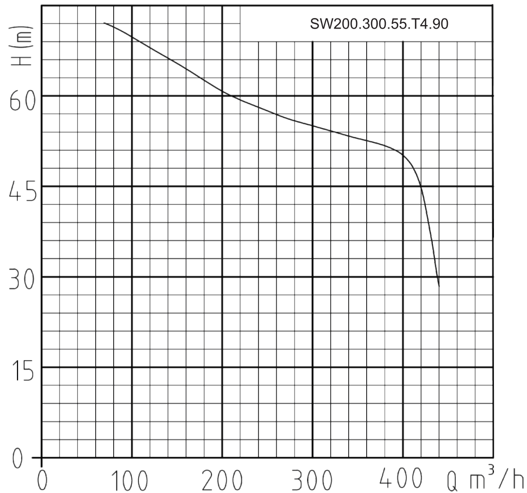
Гидравлическая кривая
