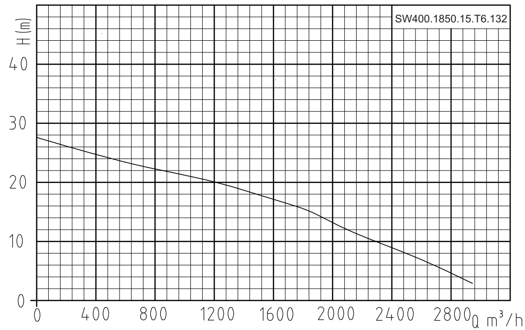
Гидравлическая кривая
