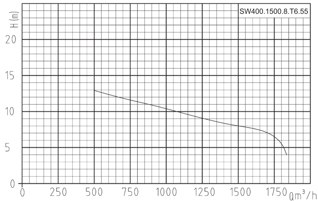
Гидравлическая кривая
