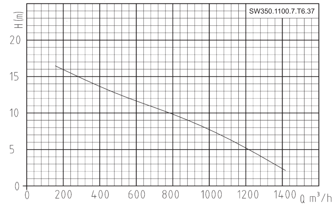
Гидравлическая кривая
