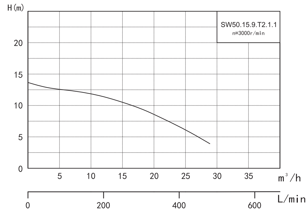
Гидравлическая кривая
