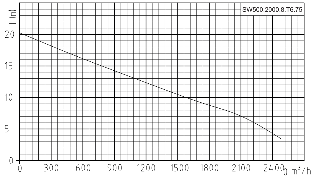
Гидравлическая кривая
