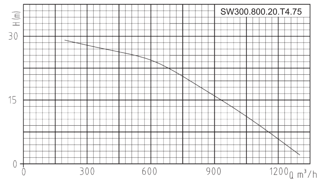
Гидравлическая кривая
