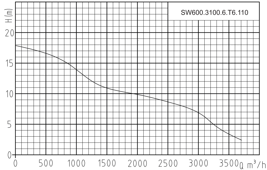
Гидравлическая кривая
