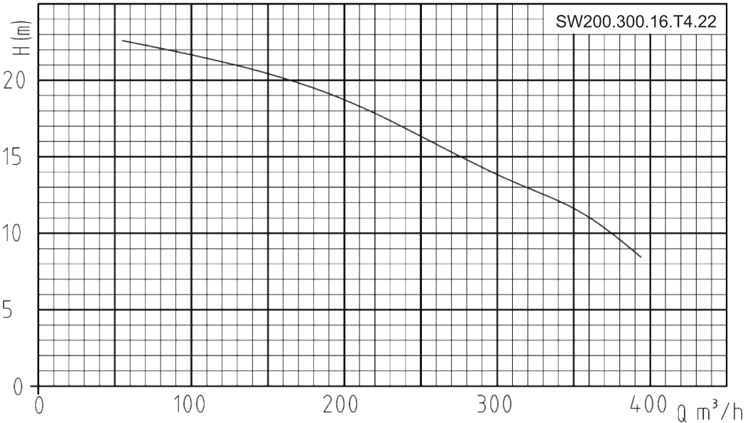
Гидравлическая кривая
