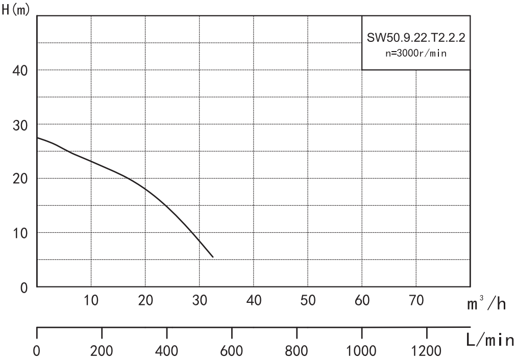
Гидравлическая кривая
