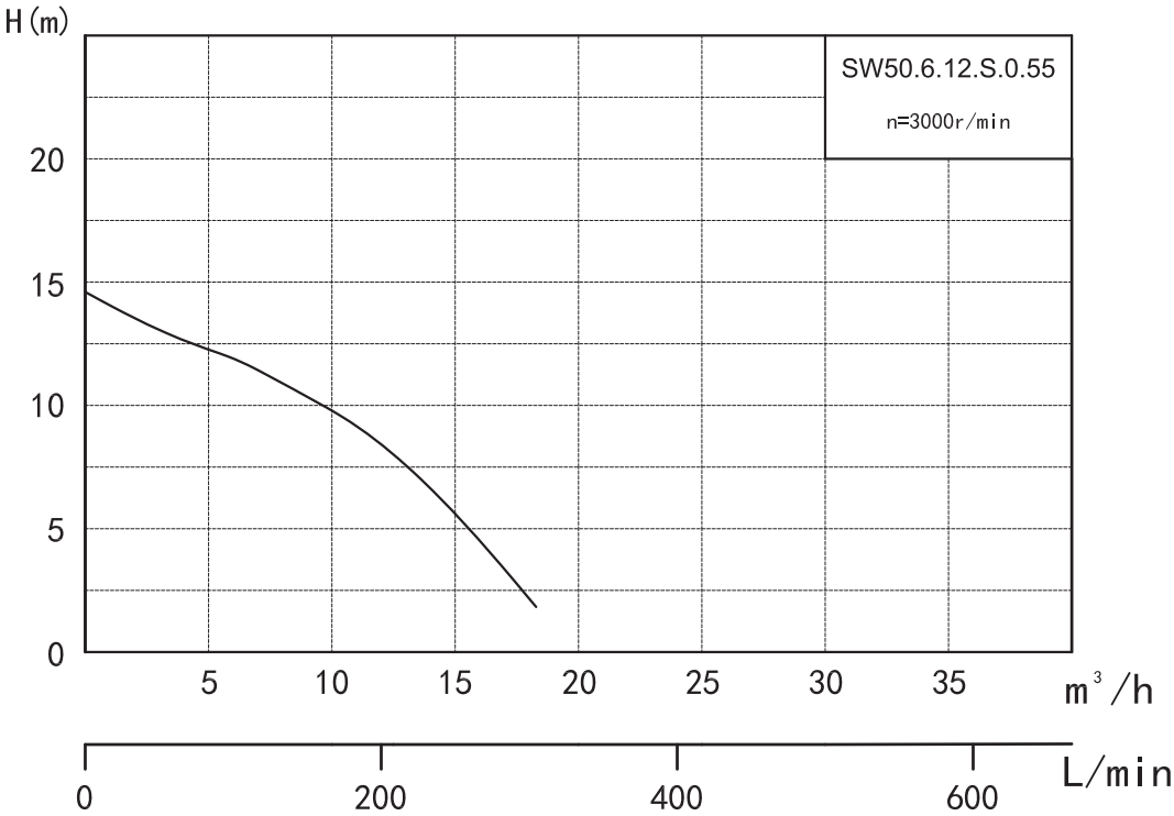
Гидравлическая кривая
