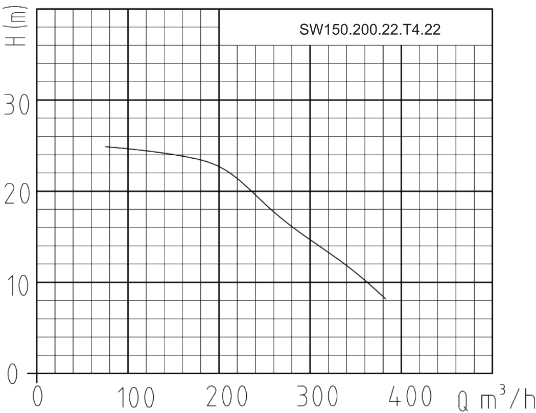
Гидравлическая кривая
