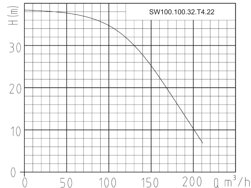
Гидравлическая кривая
