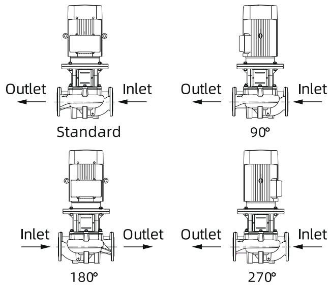
Положение распределительной коробки
