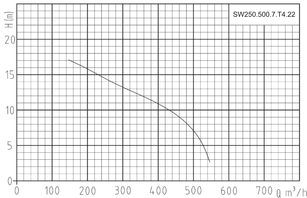
Гидравлическая кривая
