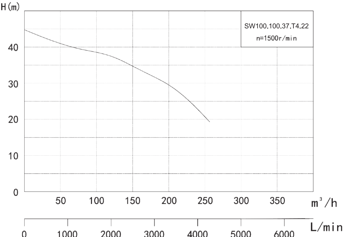
Гидравлическая кривая
