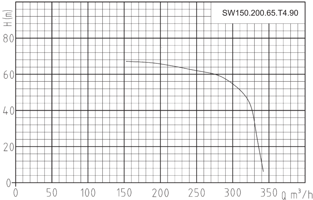
Гидравлическая кривая
