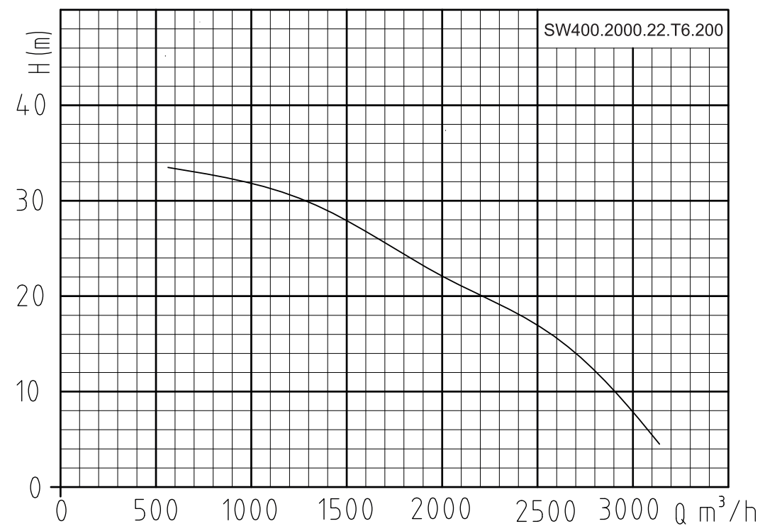
Гидравлическая кривая
