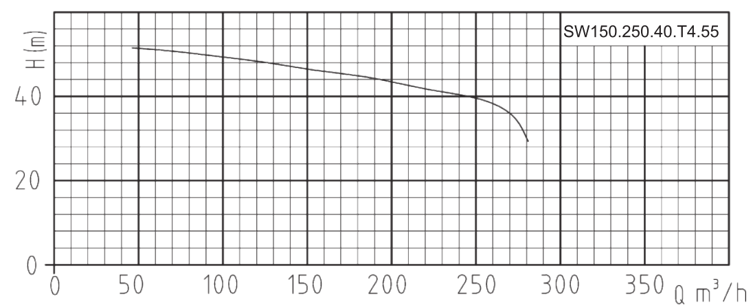
Гидравлическая кривая
