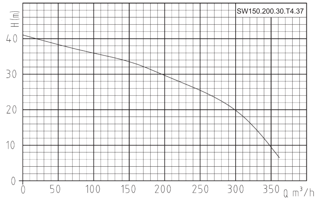
Гидравлическая кривая
