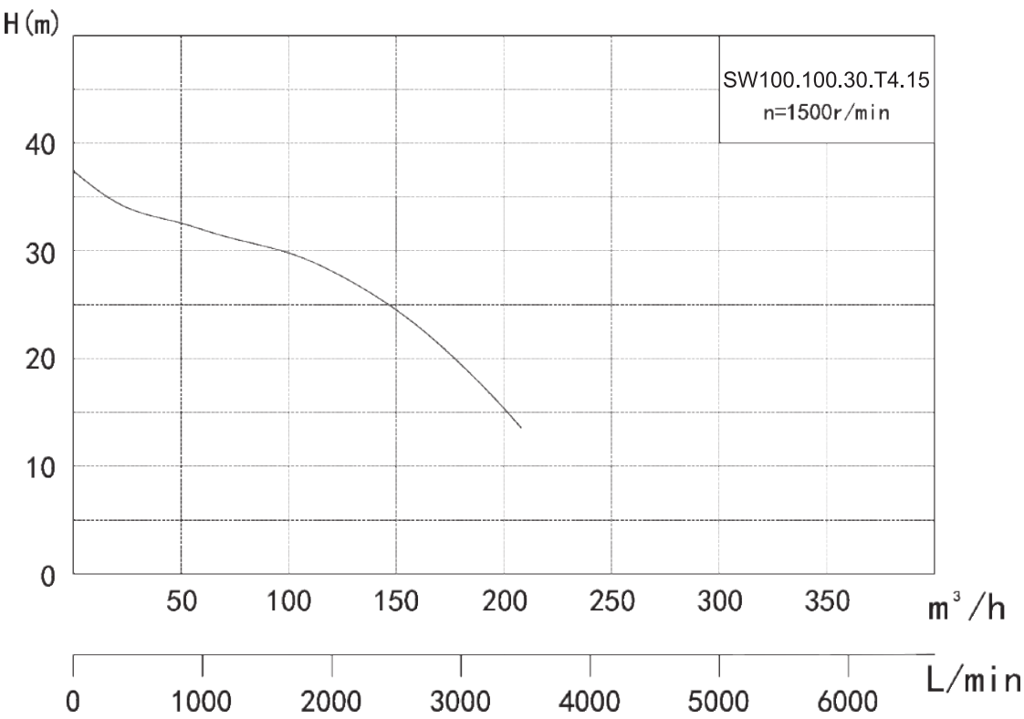
Гидравлическая кривая
