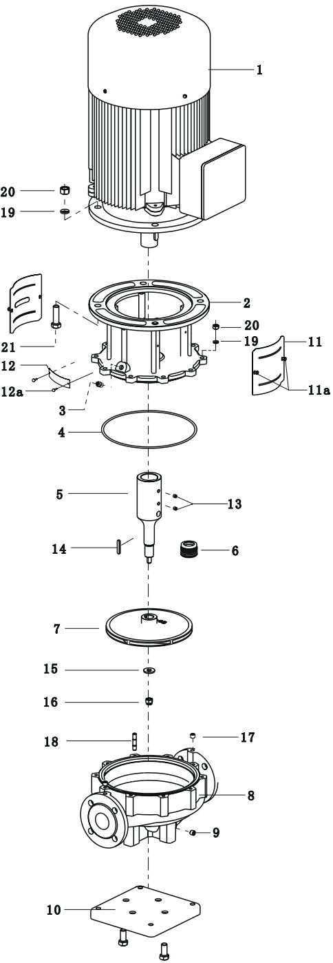
Взрыв-схема насосов INL40-INL150
