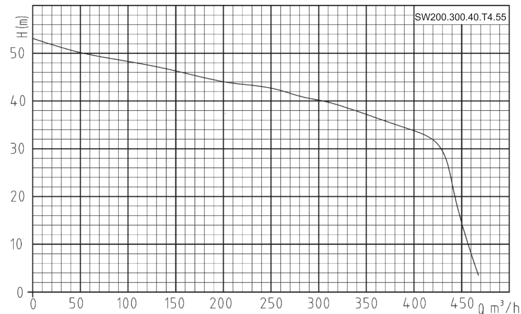
Гидравлическая кривая
