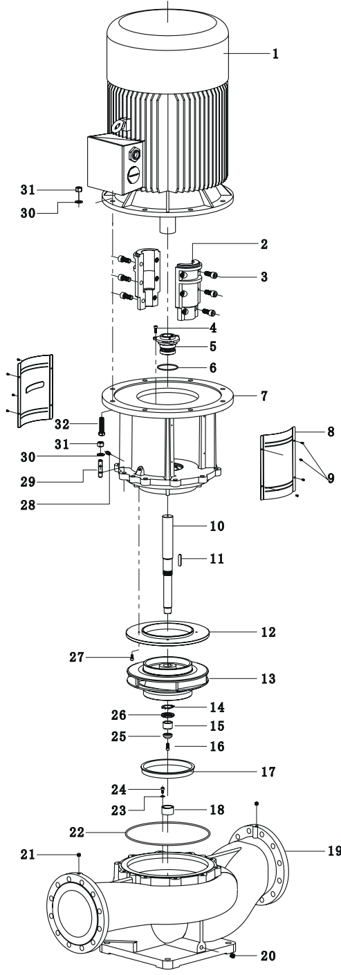
Взрыв-схема насосов INL200-INL250
