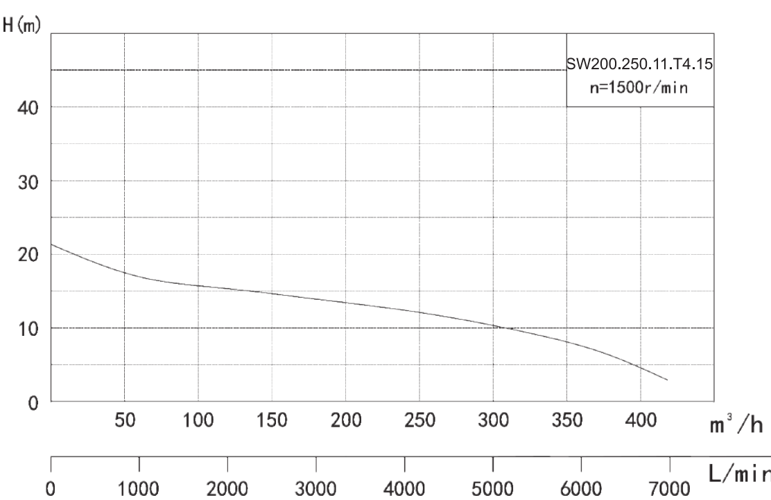
Гидравлическая кривая
