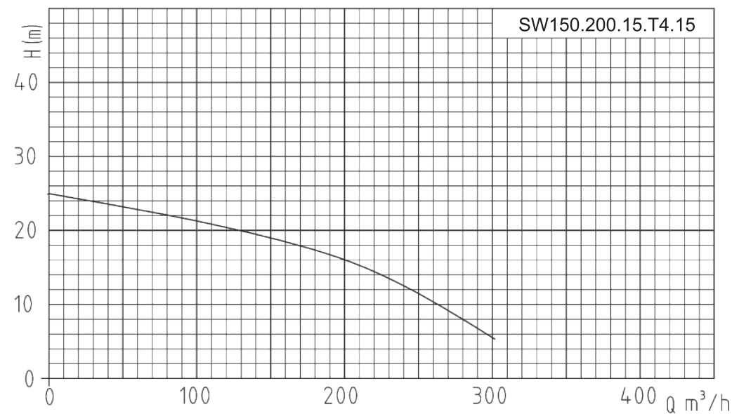
Гидравлическая кривая
