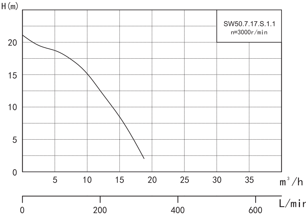
Гидравлическая кривая
