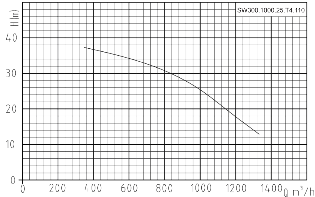
Гидравлическая кривая
