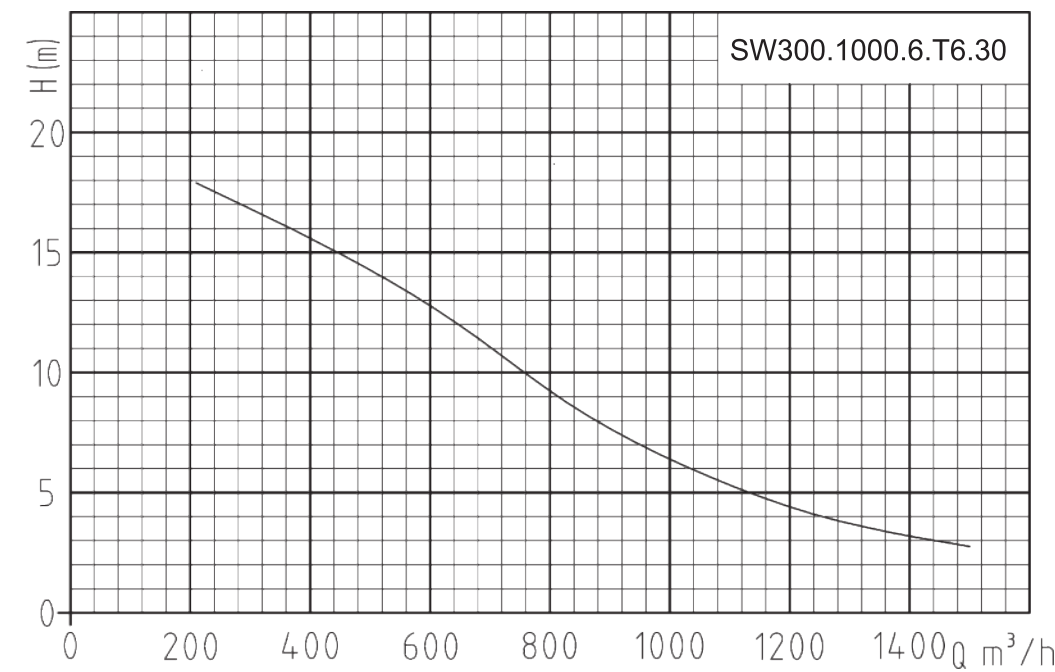
Гидравлическая кривая
