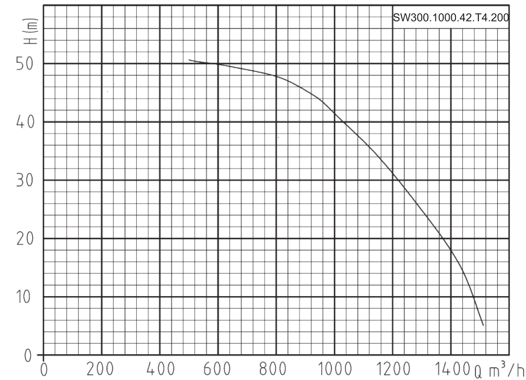
Гидравлическая кривая
