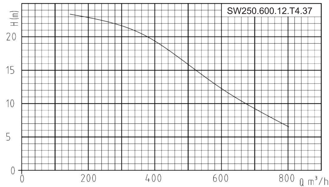
Гидравлическая кривая
