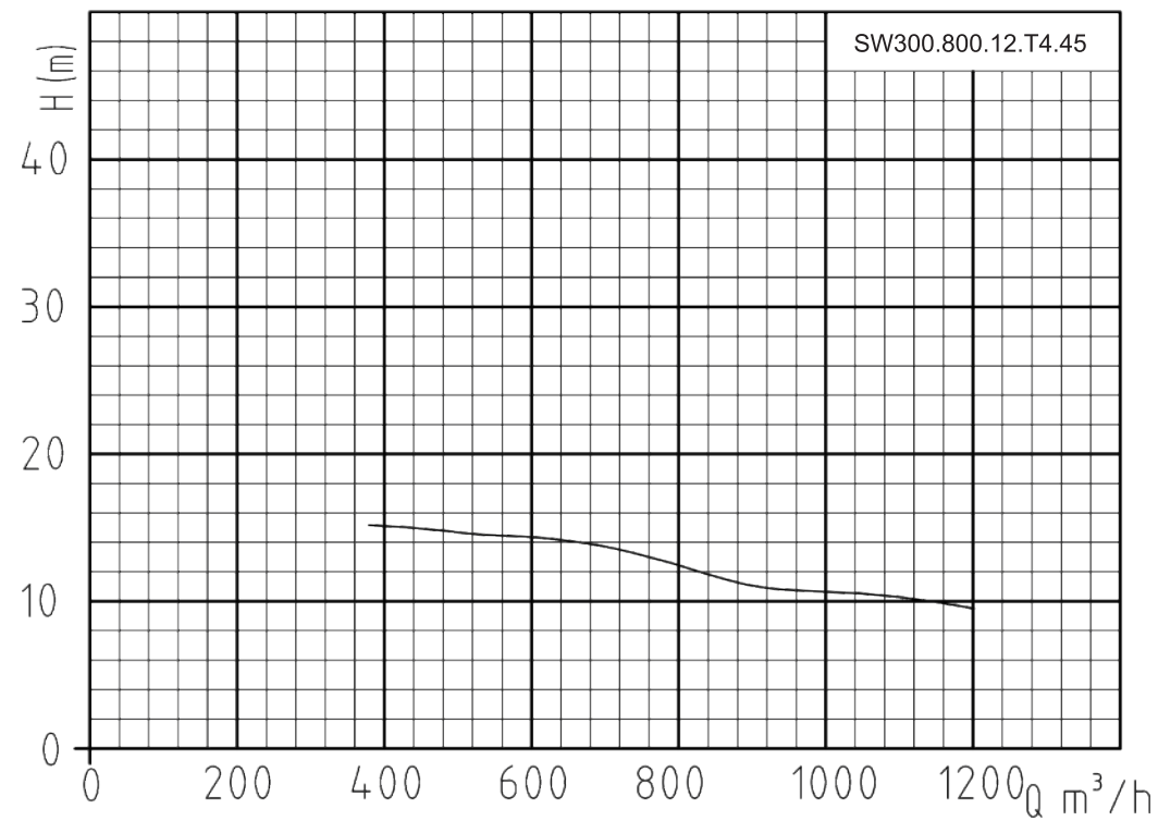
Гидравлическая кривая
