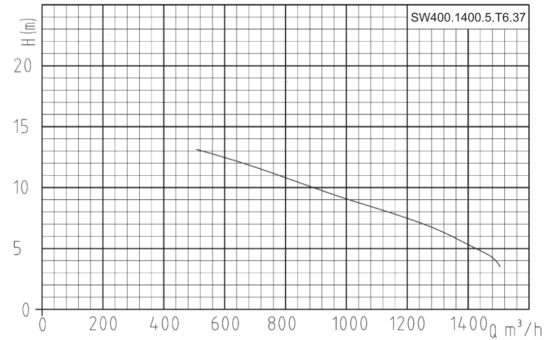
Гидравлическая кривая
