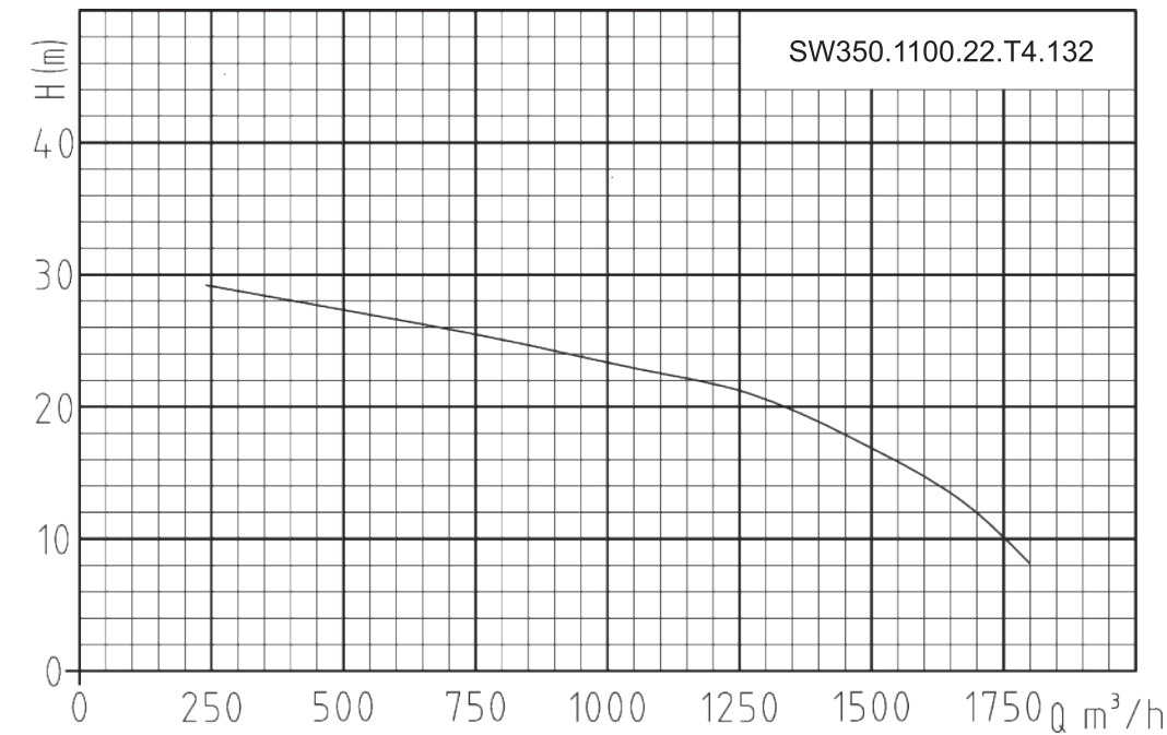
Гидравлическая кривая
