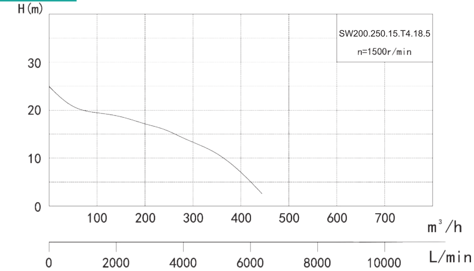
Гидравлическая кривая
