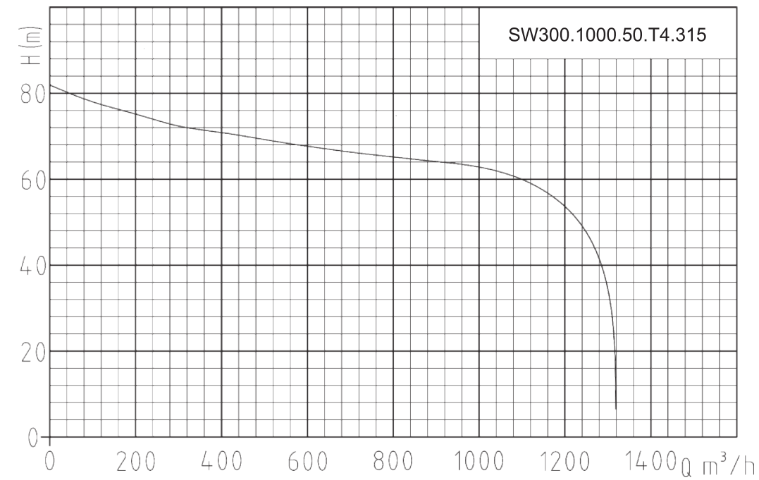
Гидравлическая кривая
