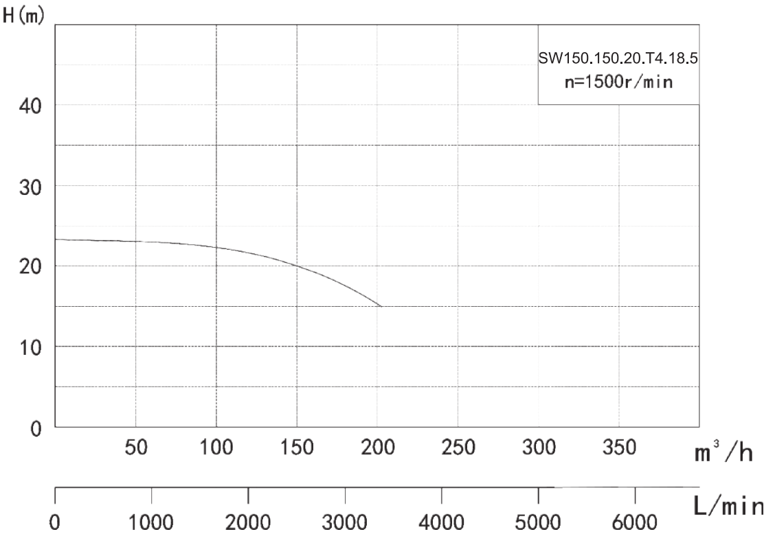
Гидравлическая кривая
