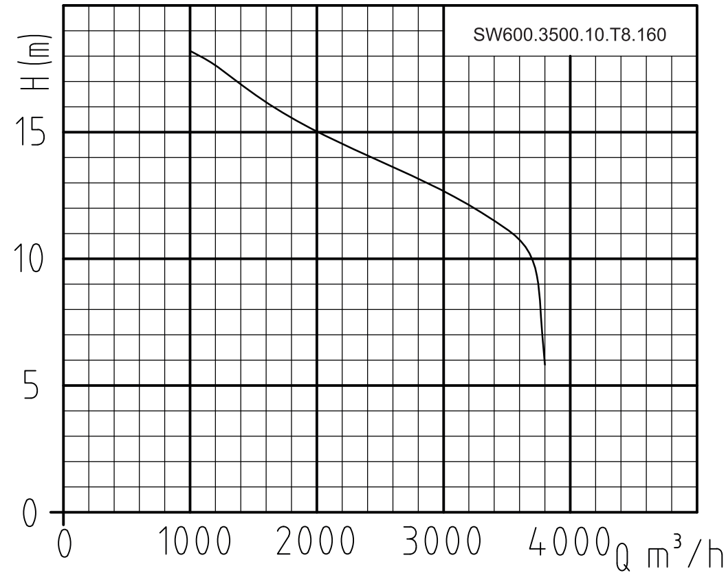
Гидравлическая кривая
