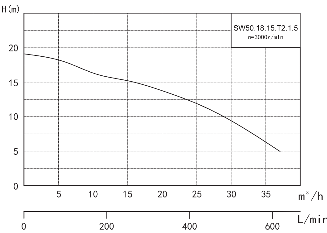
Гидравлическая кривая
