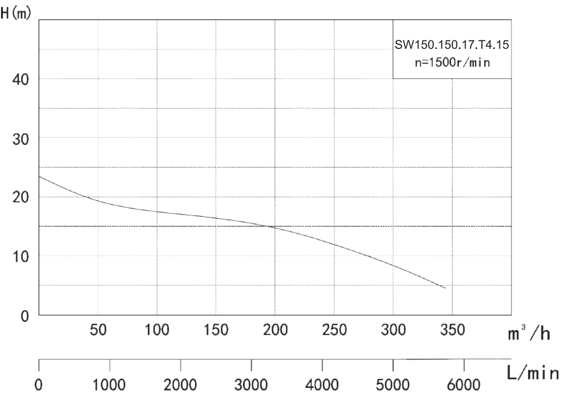
Гидравлическая кривая
