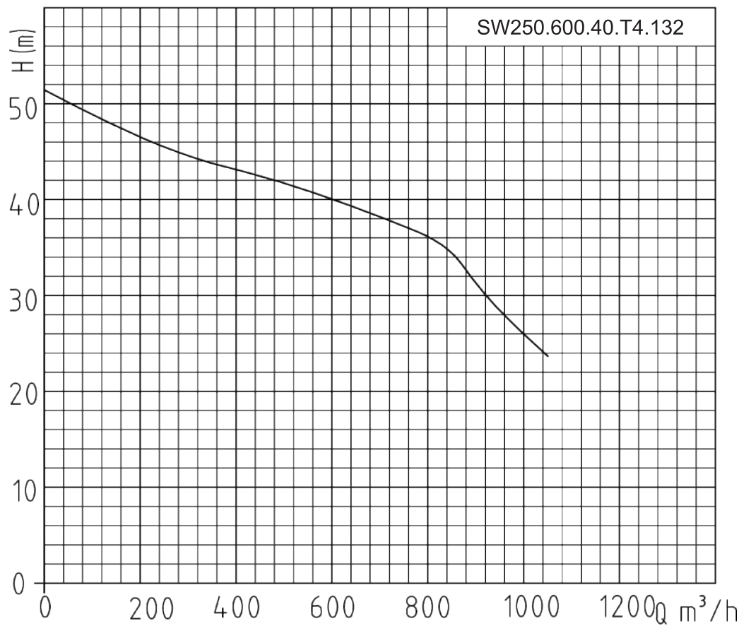
Гидравлическая кривая
