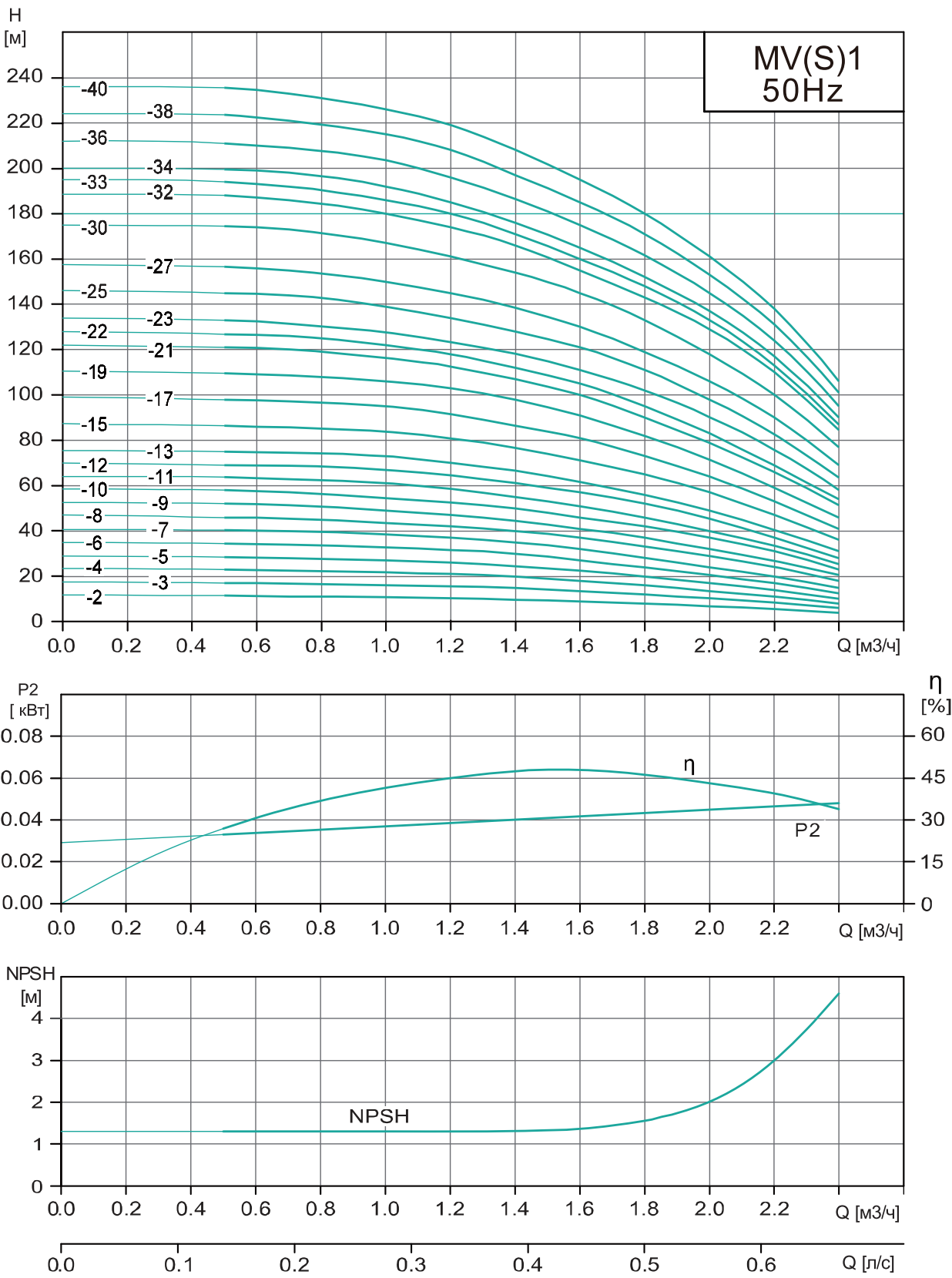
Кривая производительности MV(S)1
