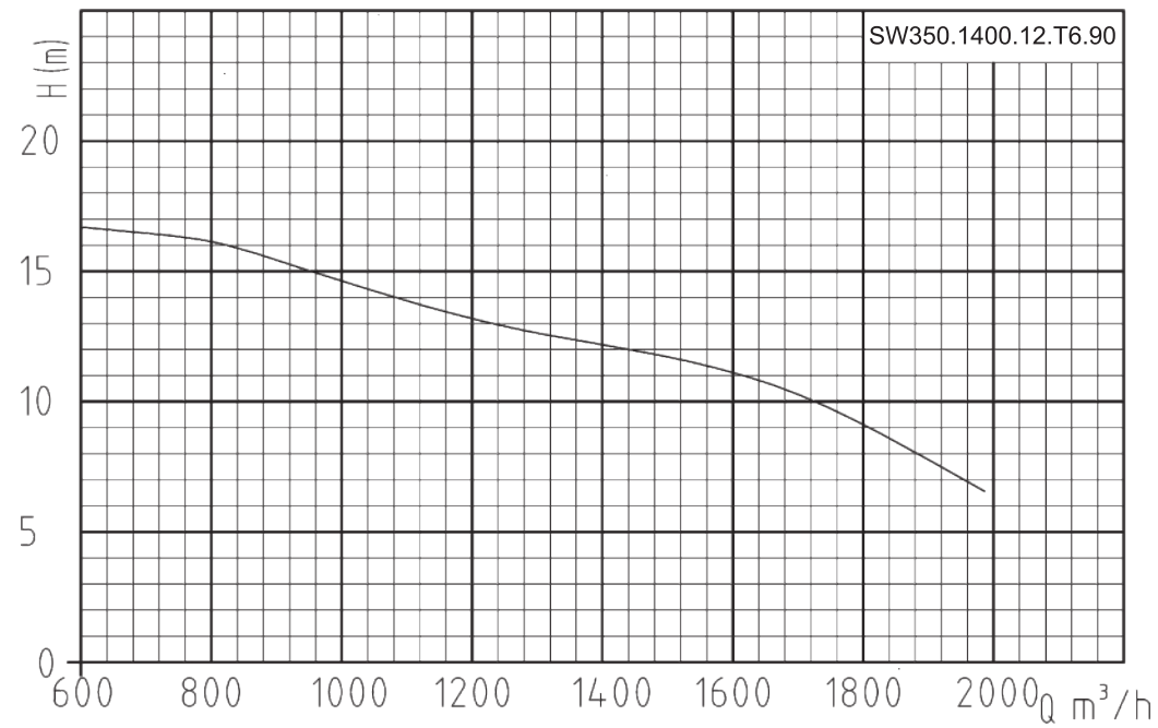
Гидравлическая кривая
