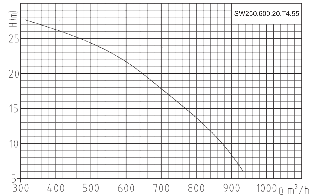
Гидравлическая кривая
