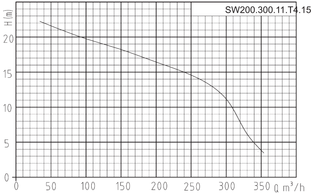
Гидравлическая кривая
