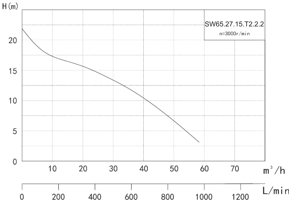
Гидравлическая кривая
