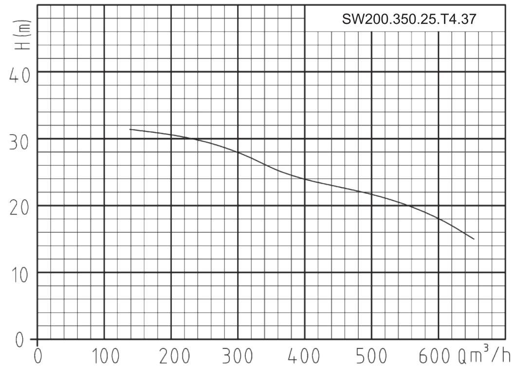
Гидравлическая кривая
