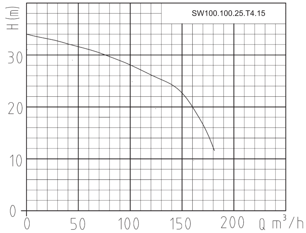
Гидравлическая кривая
