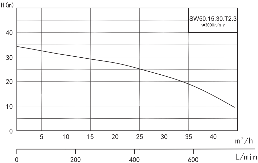
Гидравлическая кривая
