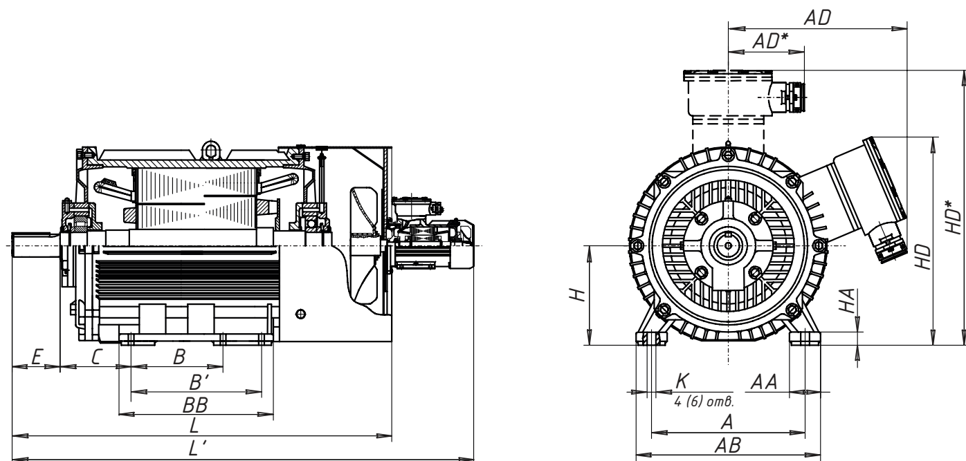
Монтажное исполнение IM 1001
