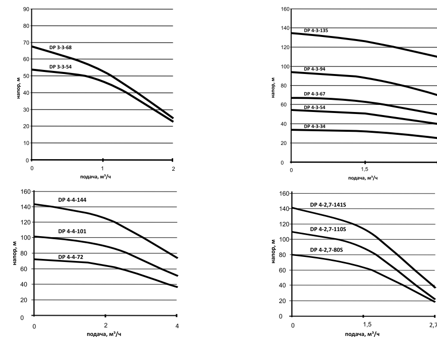
Рисунок 1. Напорно-расходные характеристики насоса
