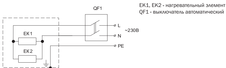
Рис. 2. Обогреватель OTGON 2.0-ИH
