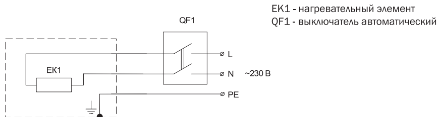
Рис. 2. Обогреватель OTGON 2.0-ИH
