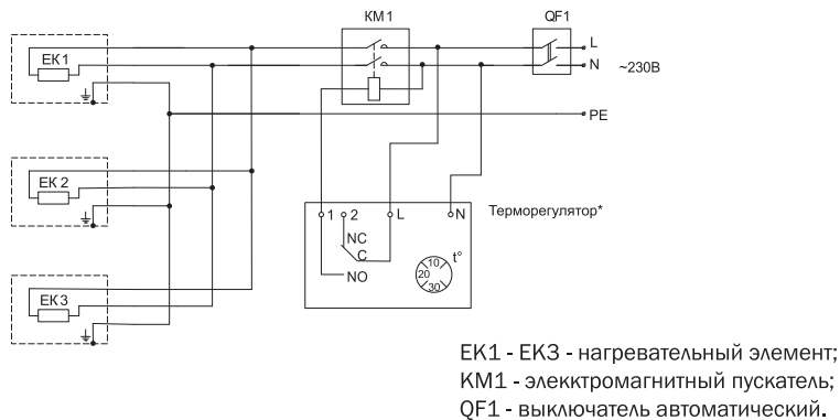
Рис. 3. Обогреватель OTGON 0.8-ИH; OTGON 1.0-ИH, обогреватель OTGON 2.0-ИH подключается аналогично
