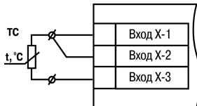
Рисунок 6.7 – Трехпроводная схема подключения ТС
