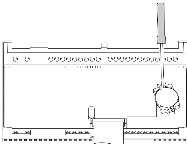
Рисунок 9.2 – Замена батарейки
