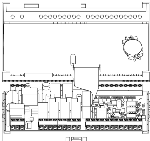
Рисунок 9.1 – Открытие корпуса
