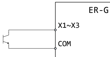
Б) Сигнал типа «открытый коллектор»
