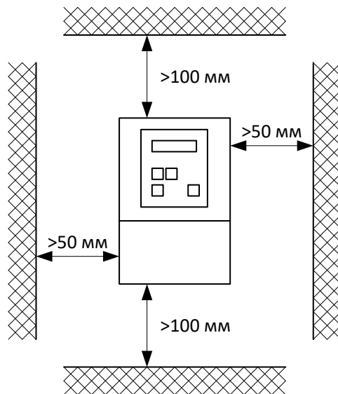
Рисунок 3 – Установка ПЧ
