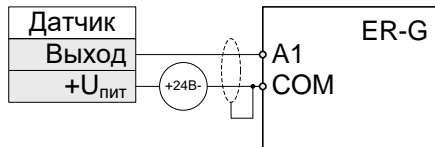
Рисунок 8 – Типовые схемы подключения аналоговых входов A1, A2
