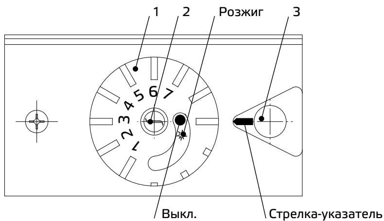
Рисунок 2 — Блок газовый
