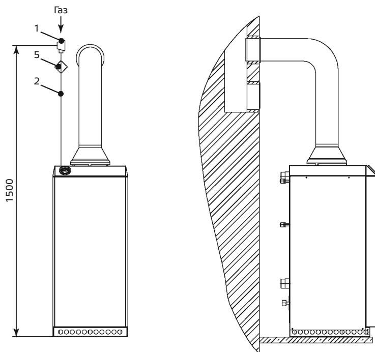
Рисунок 7 — Подключение аппарата к дымоходу и газопроводу
