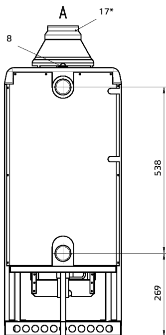
Рисунок 1 — Аппарат отопительный газовый бытовой одноконтурный
