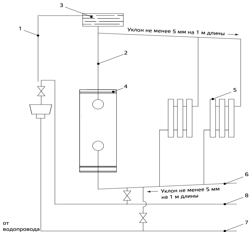
Рисунок 4 — Примерная открытая схема системы отопления
