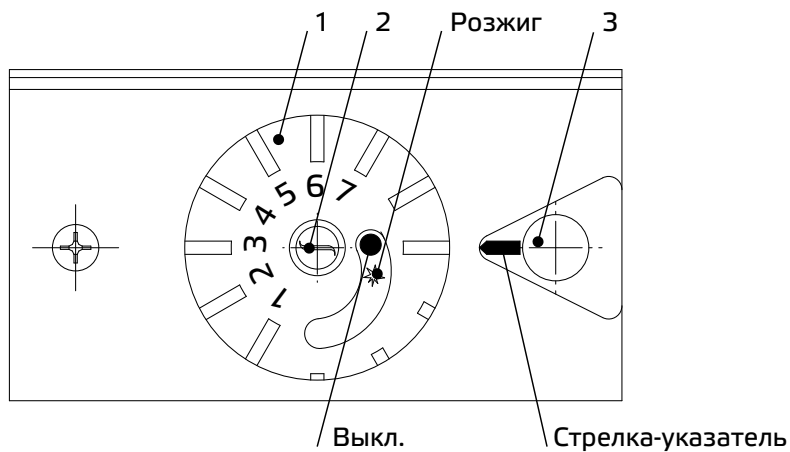
Рисунок 2 — Блок газовый
