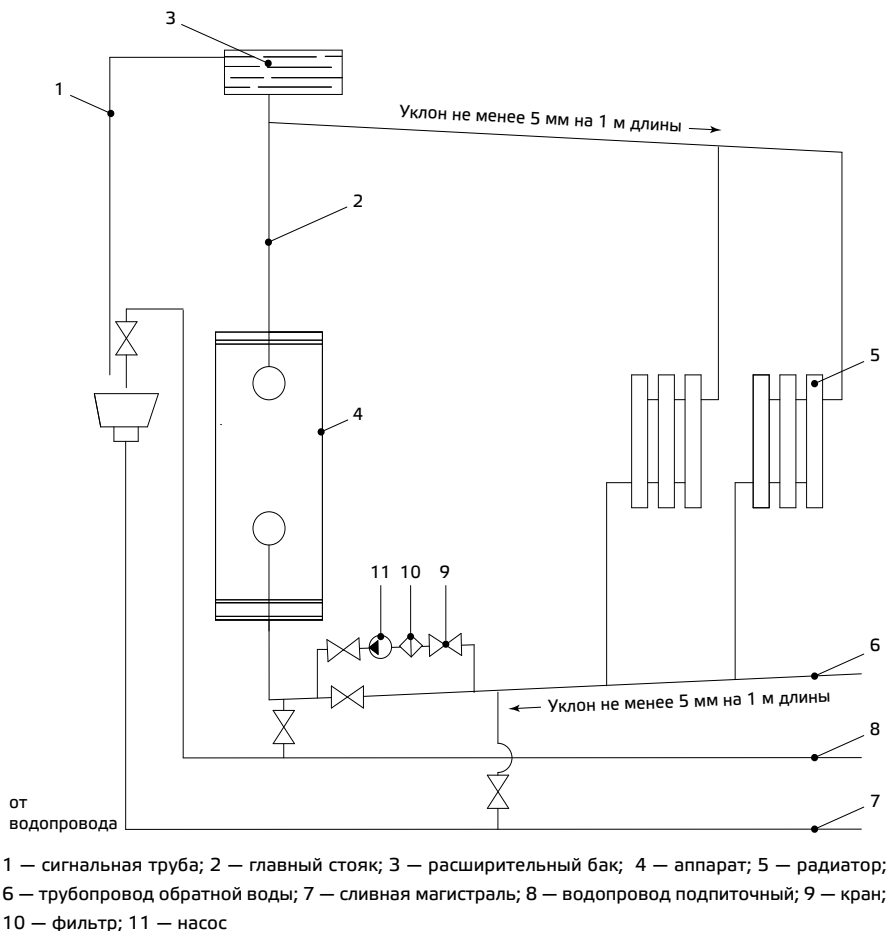
Рисунок 4 — Примерная открытая схема системы отопления с использованием насоса
