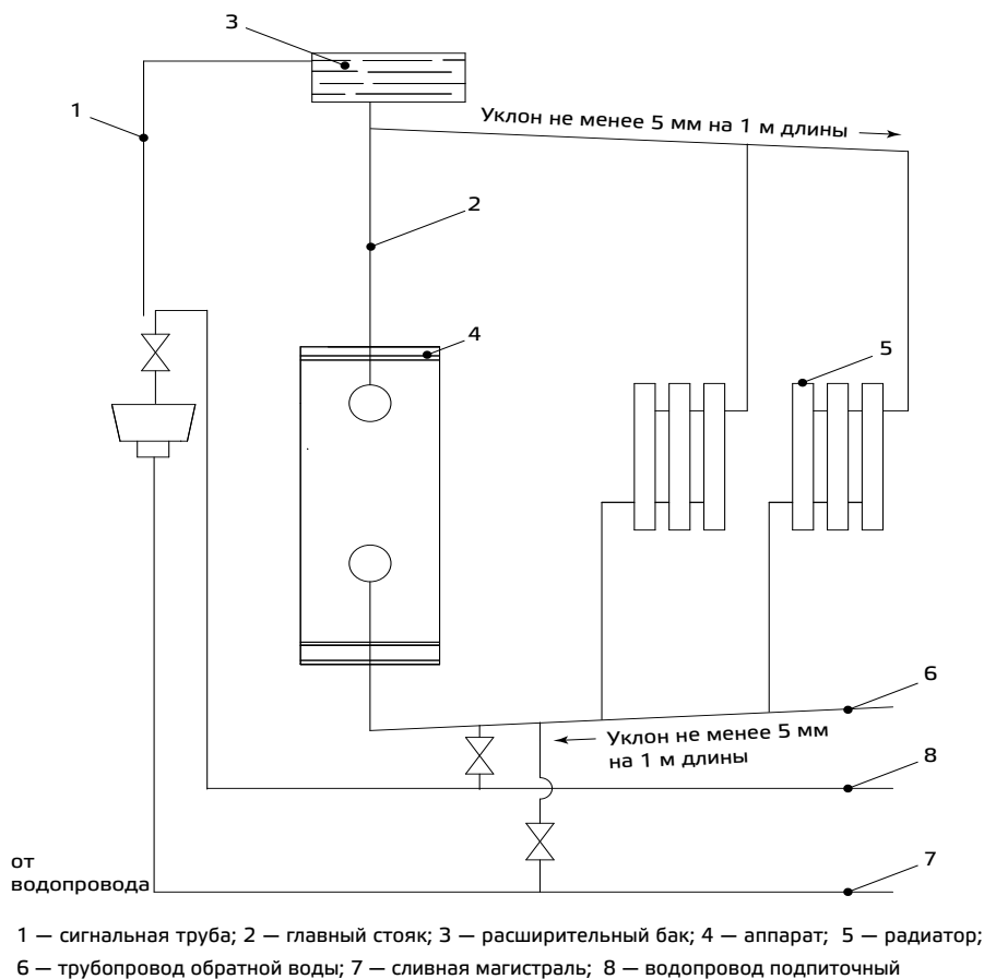
Рисунок 3 — Примерная открытая схема системы отопления
