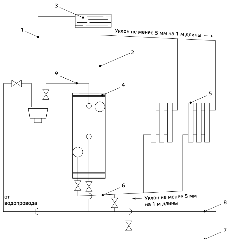
1 — сигнальная труба; 2 — главный стояк; 3 — расширительный бак; 4 — аппарат; 5 — радиатор; 6 — трубопровод обратной воды; 7 — сливная магистраль; 8 — водопровод подпиточный; 9 — трубопровод горячей воды
