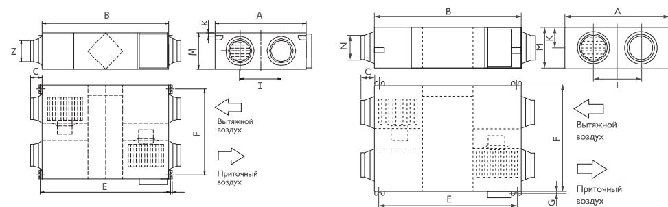
Модель RCS-350-U
