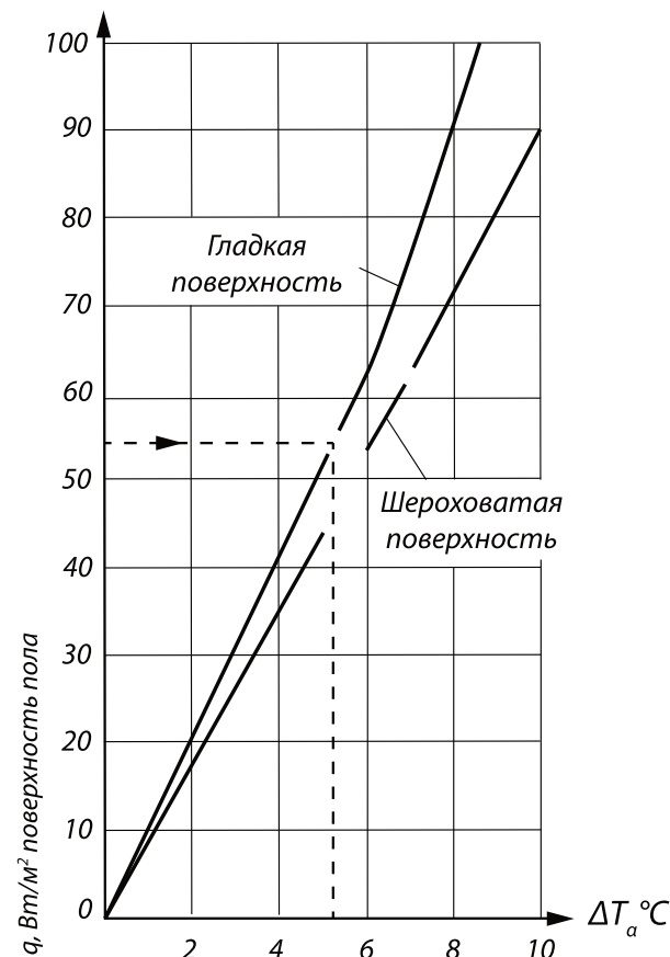
Рисунок 58. График теплоотдачи поверхности пола.
