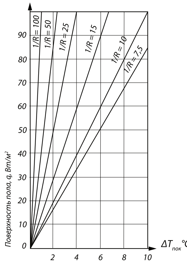
Рисунок 59. График понижения температуры через покрытие пола.
