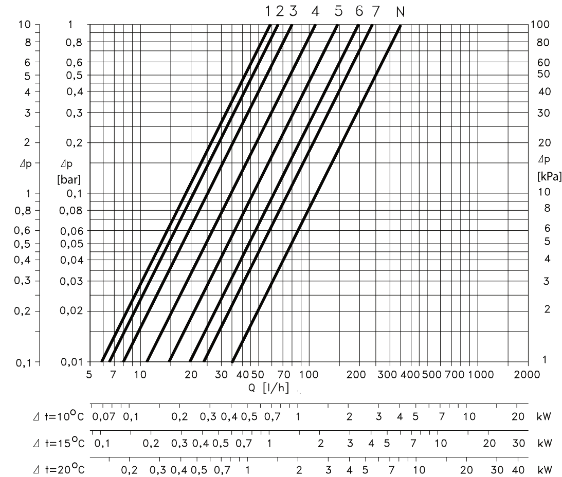
Диаграмма для определения предварительной настройки клапана RA-U 013G1383 с установленным термоэлементом серии RA 2000 при Xp=2°C
