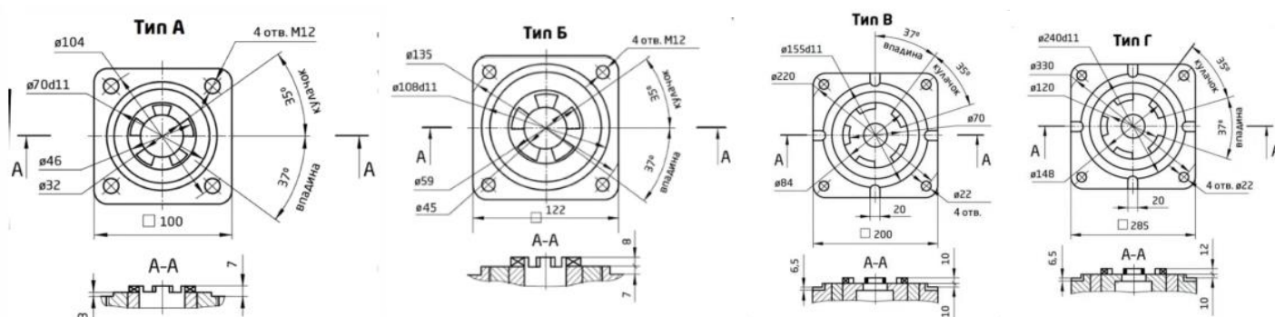
Рис.4. Присоединительные размеры верхнего фланца (ОСТ) задвижки 30с941нж под электропривод.
