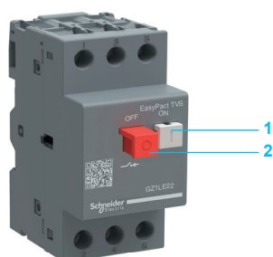
GZ1LE
