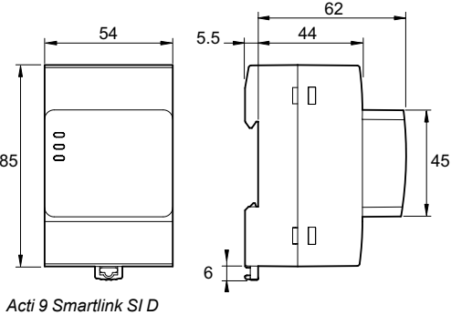
Acti 9 Smartlink SI D
