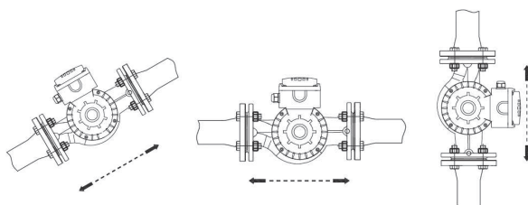
Рис. 17 Возможные положения клеммной коробки
