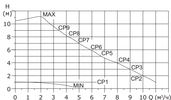
Рис. 39 Кривые режима управления с постоянным значением давления.
