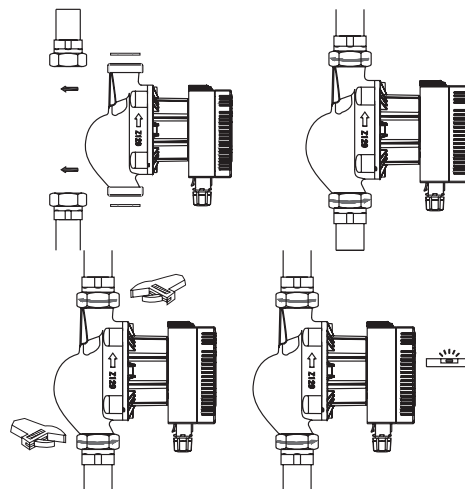
Рис. 35 Монтаж насоса
