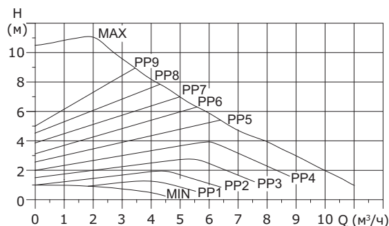
Рис. 38 Кривые режима управления пропорционального изменения давления
