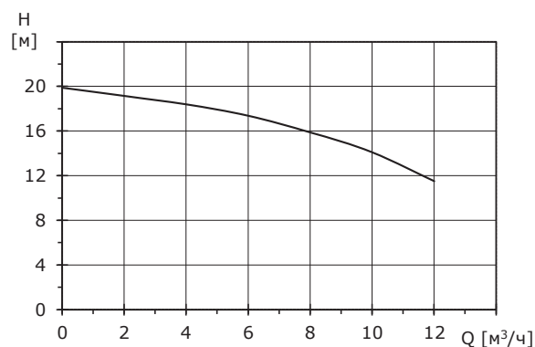
BASIC 25-20 230
