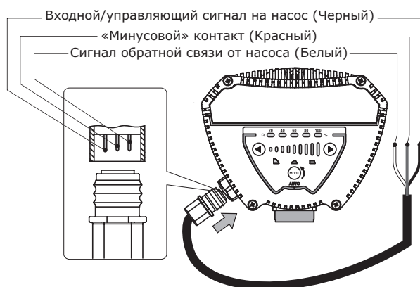
Рис. 42 Схема подключения ШИМ-сигнала
