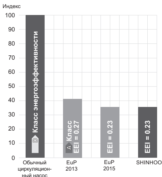
Рис. 2 Индекс энергопотребления
