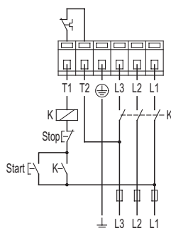
Рис. 19 Трехфазный без нейтрального провода
