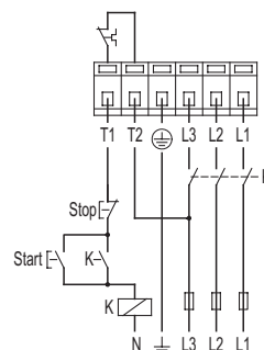
Рис. 20 Трехфазный с нейтральным проводом
