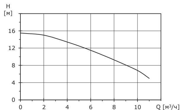
BASIC 25-16 230
