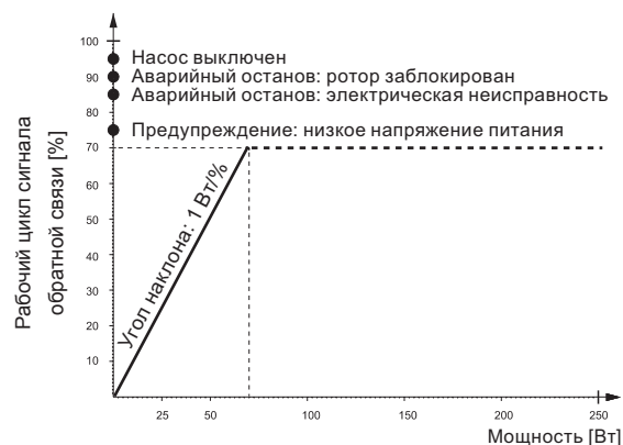
Рис. 28 Профиль ШИМ-сигнала обратной связи
