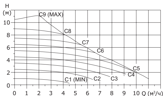
Рис. 40 Кривые режима управления при фиксированной частоте вращения
