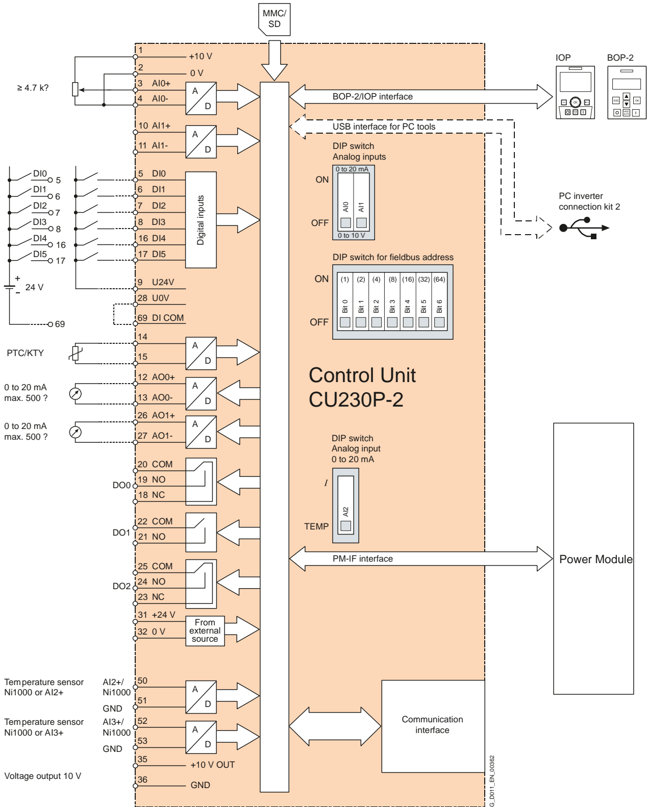
Диаграмма соединений управляющего модуля CU230P-2 ВТ.
