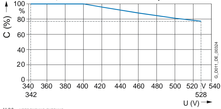
Снижение мощности в зависимости от напряжения питания
