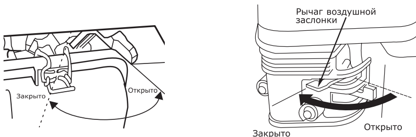
Рис. 15. Рычаг привода воздушной заслонки
