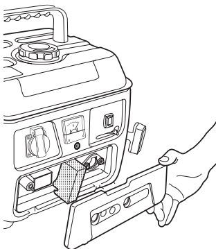
Фильтрующий элемент
