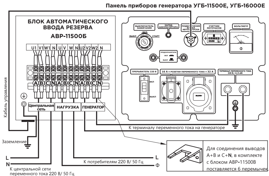
Рис. 21. Рекомендуемая схема подключения резерва АВР-11500Б (3 фазы)
