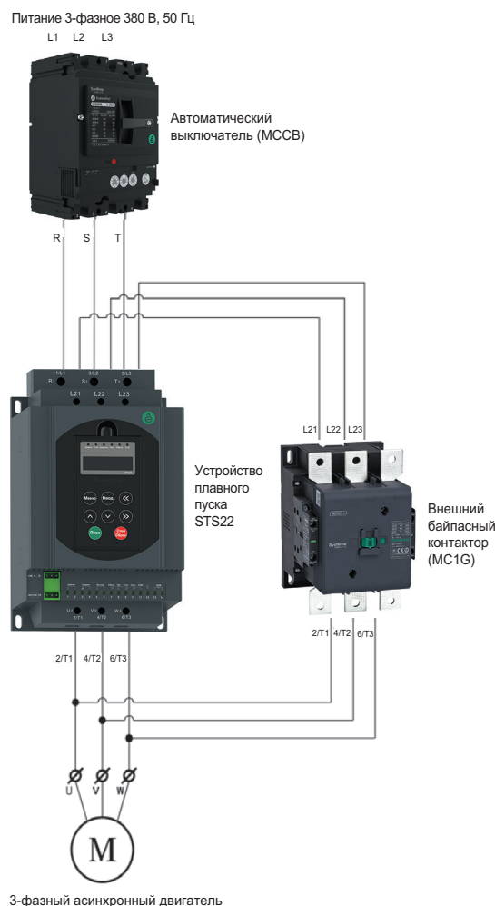
Схема подключения
