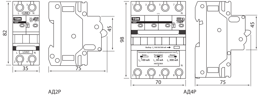
Рисунок 2. Габаритные и установочные размеры, мм
