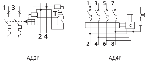
Рисунок 3. Схемы электрические принципиальные
