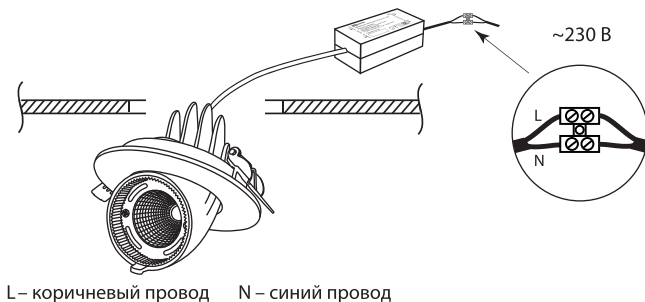
Рисунок 2. Подключение светильника с драйвером к электрической сети
