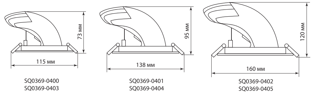
Рисунок 1. Габаритные размеры светильников, мм
