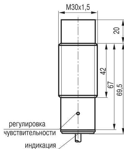
Габаритный чертеж
