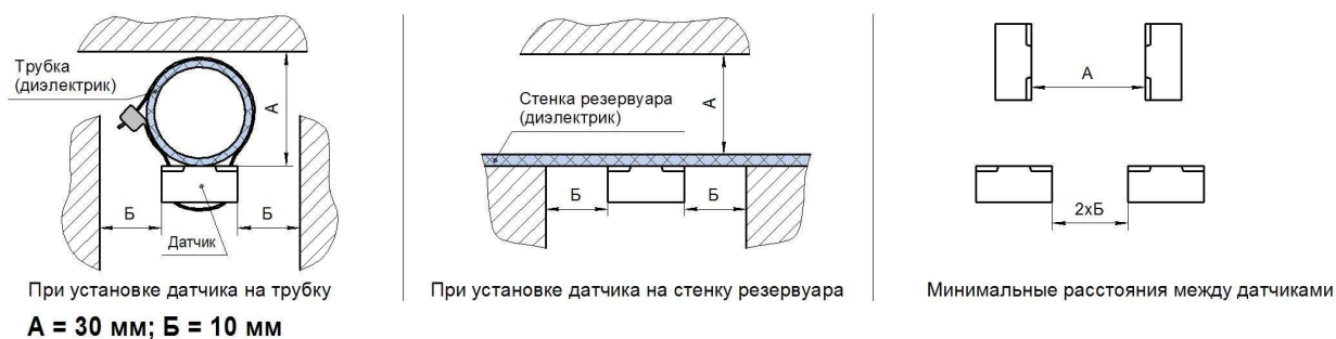
Рис.1 - Минимальные расстояния от датчика до окружающих объектов и между датчиками
